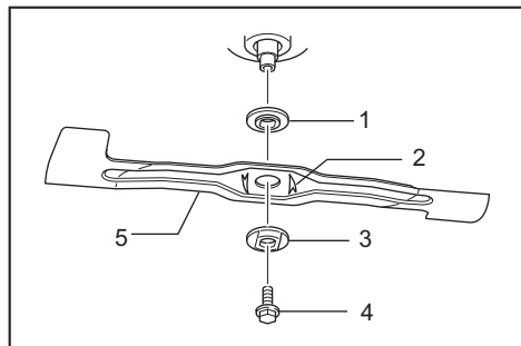
► 1. Brida interior 2. Flecha de dirección de giro 3. Brida exterior 4. Perno 5. Cuchilla de la cortadora de césped
